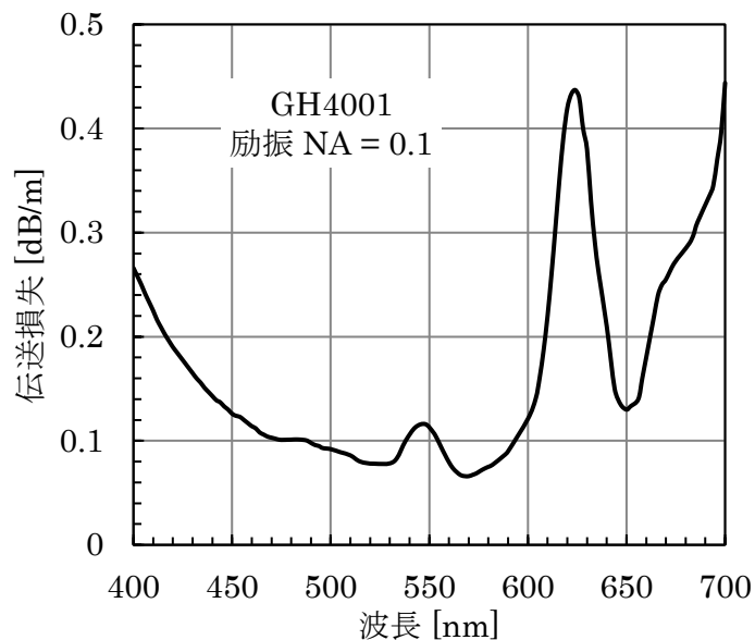
図 1-1 エスカプレミア ® ケーブル GH-4001 の伝送損失スペクトル
