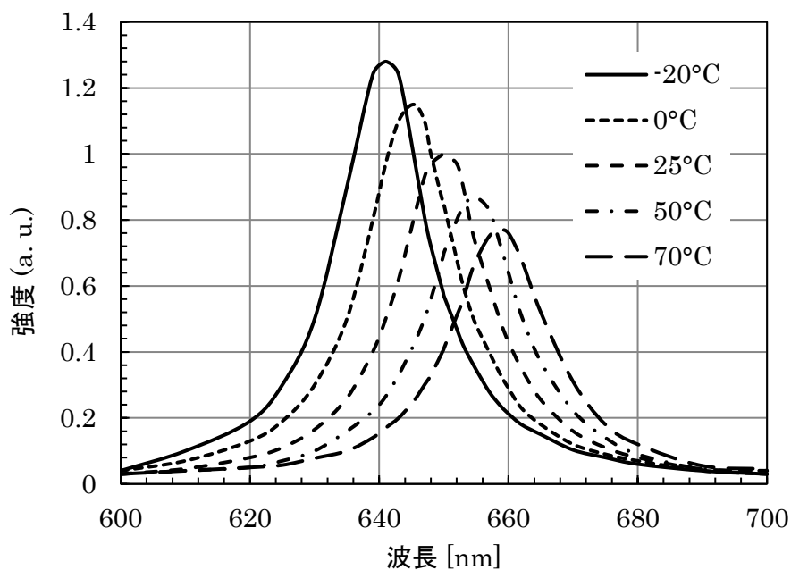
図 2-4 発光スペクトルの温度依存性
