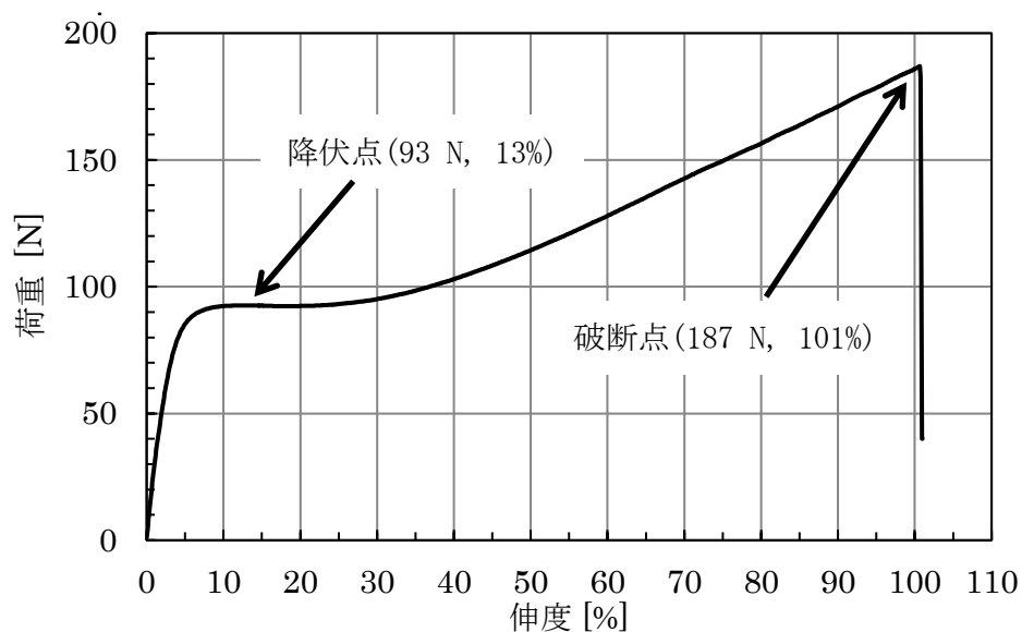
図 4-3 エスカプレミア ® ケーブル GH-4001 の引張特性
