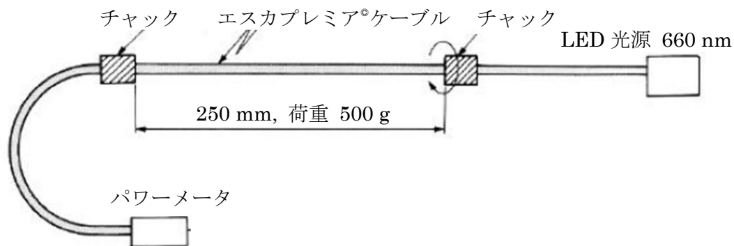
図 4-6-b 連続捻回試験の概略図
