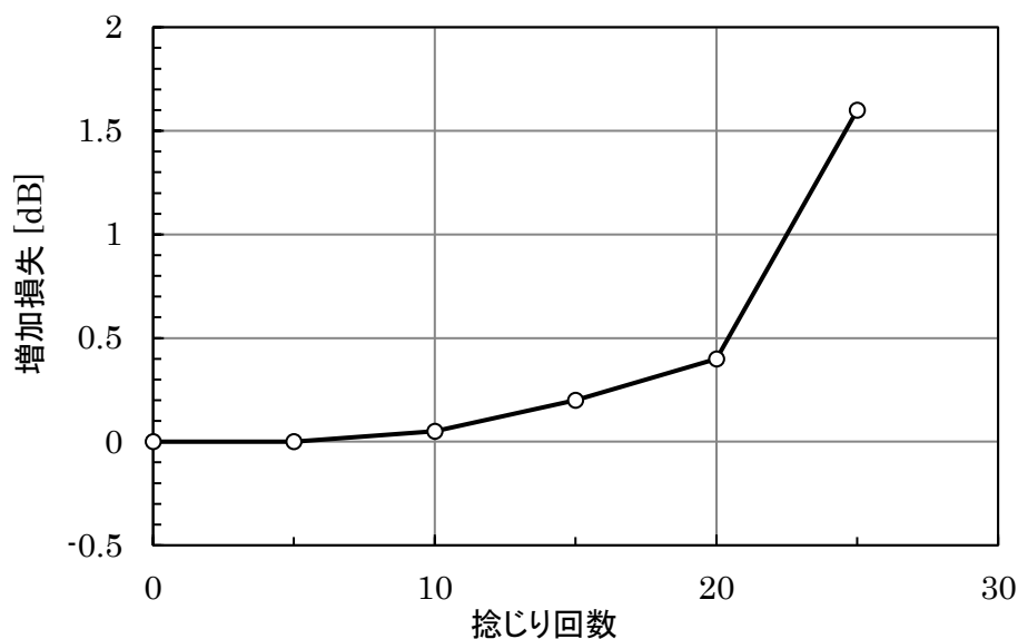
図 4-6-a エスカプレミア ® ケーブル GH-4001 における連続捻回試験後の増加損失
